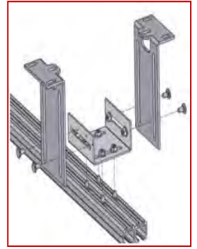
Fixation au plafond dans le refoulement
